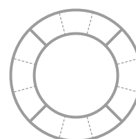
1360x362x741/1087/1433 Ø внутренний 1184 Ø внешний 1908
