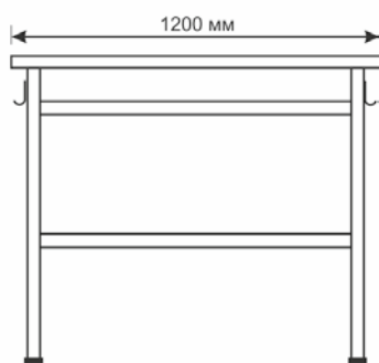
СТОЛ УЧЕНИЧЕСКИЙ ДВУХМЕСТНЫЙ
