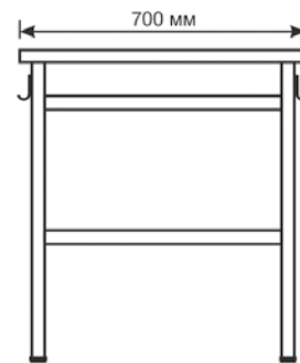
СТОЛ УЧЕНИЧЕСКИЙ ОДНОМЕСТНЫЙ
